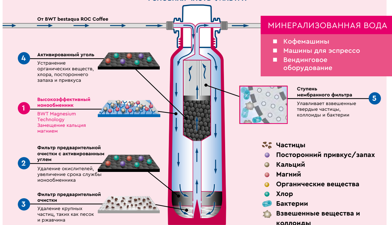
BWT BESTAQUA PREMIUM FILTER ФИЛЬТР
