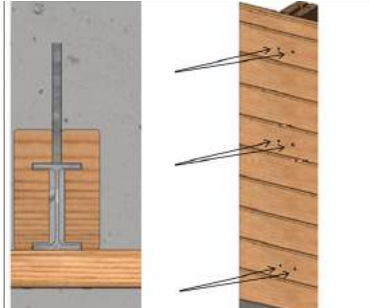
Рисунок 12 – Установка монтажных профилей опорных стоек
