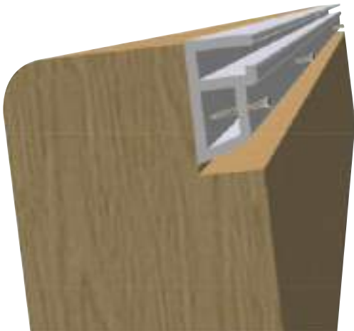
Рисунок 30 – Установка рейки
