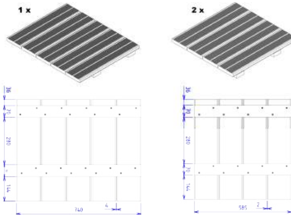
Рисунок 52 – Сборка решетки
